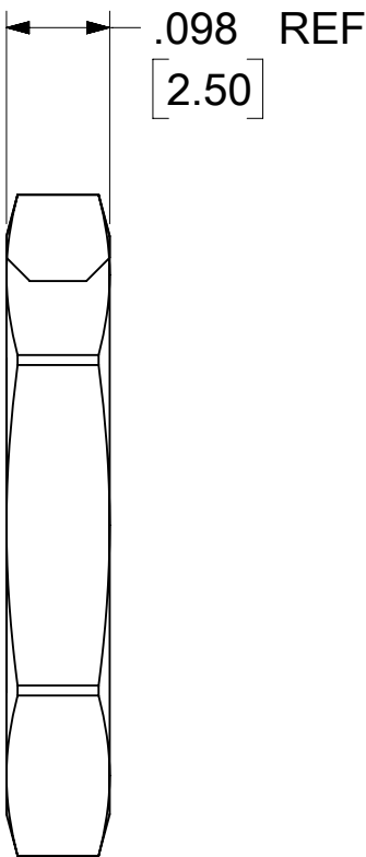
JAM NUT
